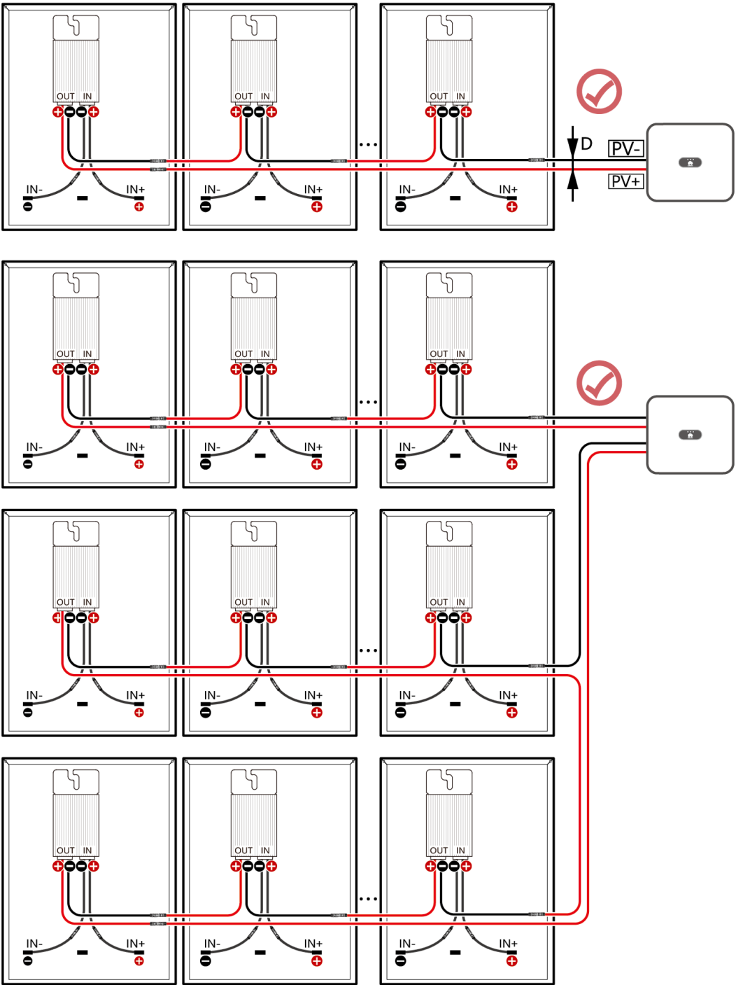
Abbildung 3-7 Erforderliche Verkabelung
